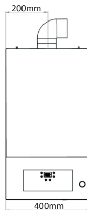
Figure 6 c (28-35 kW Davanti)
