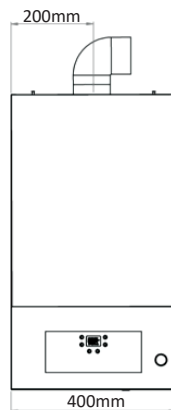
Figura 6 c (28-35 kW frente)
