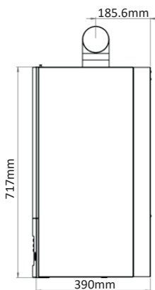
Figure 6 c (28-35 kW Lato)
