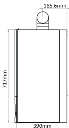
Figure 6 c (28-35 kW côté)
