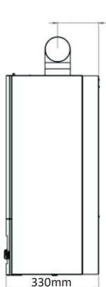
Figure 6 b (24 kW côté)
